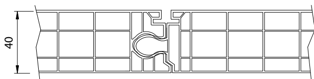
Szczegół połączenia dwóch paneli
